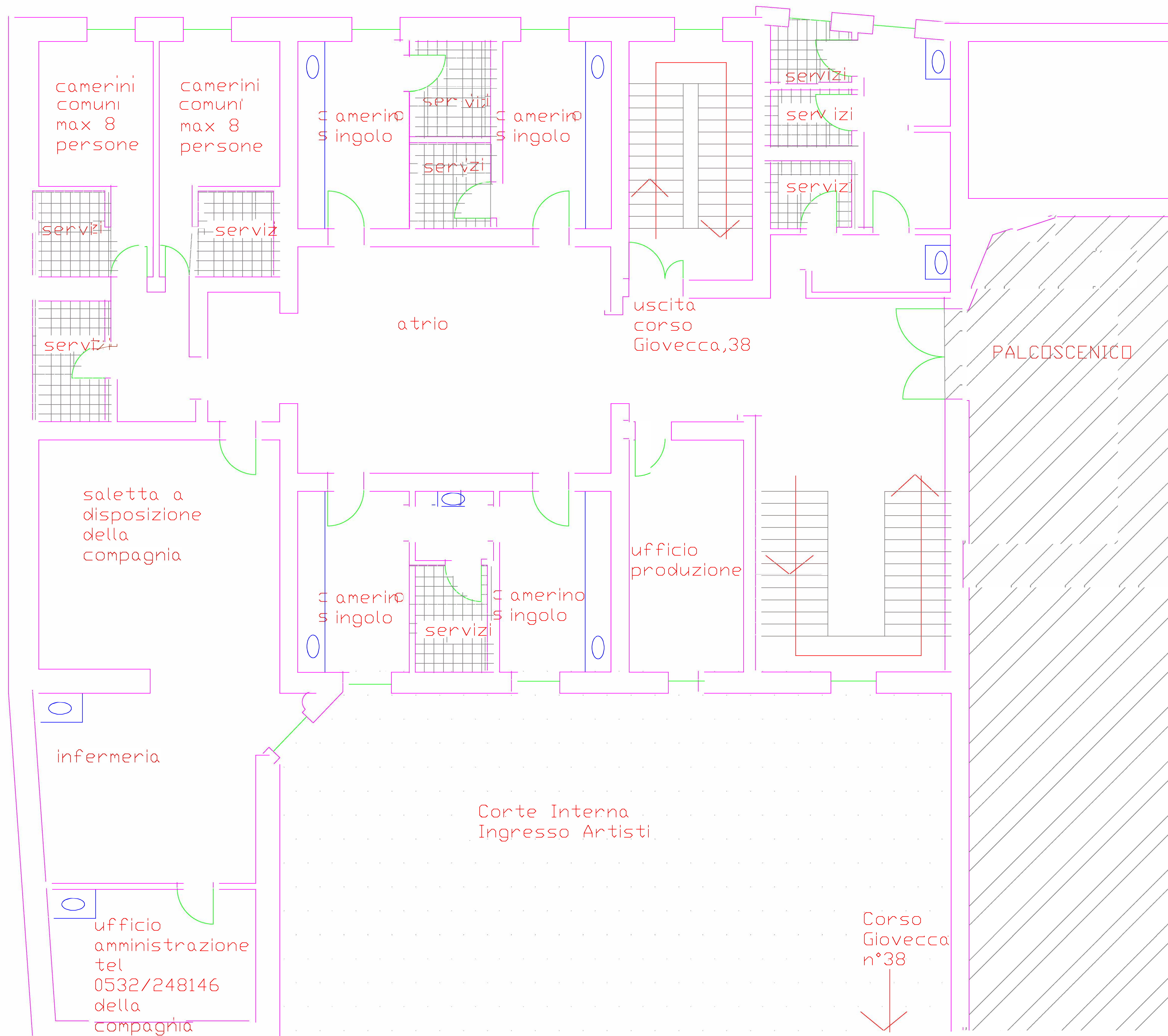
Teatro Comunale di Ferrara-Planimetria Camerini Primo Piano
