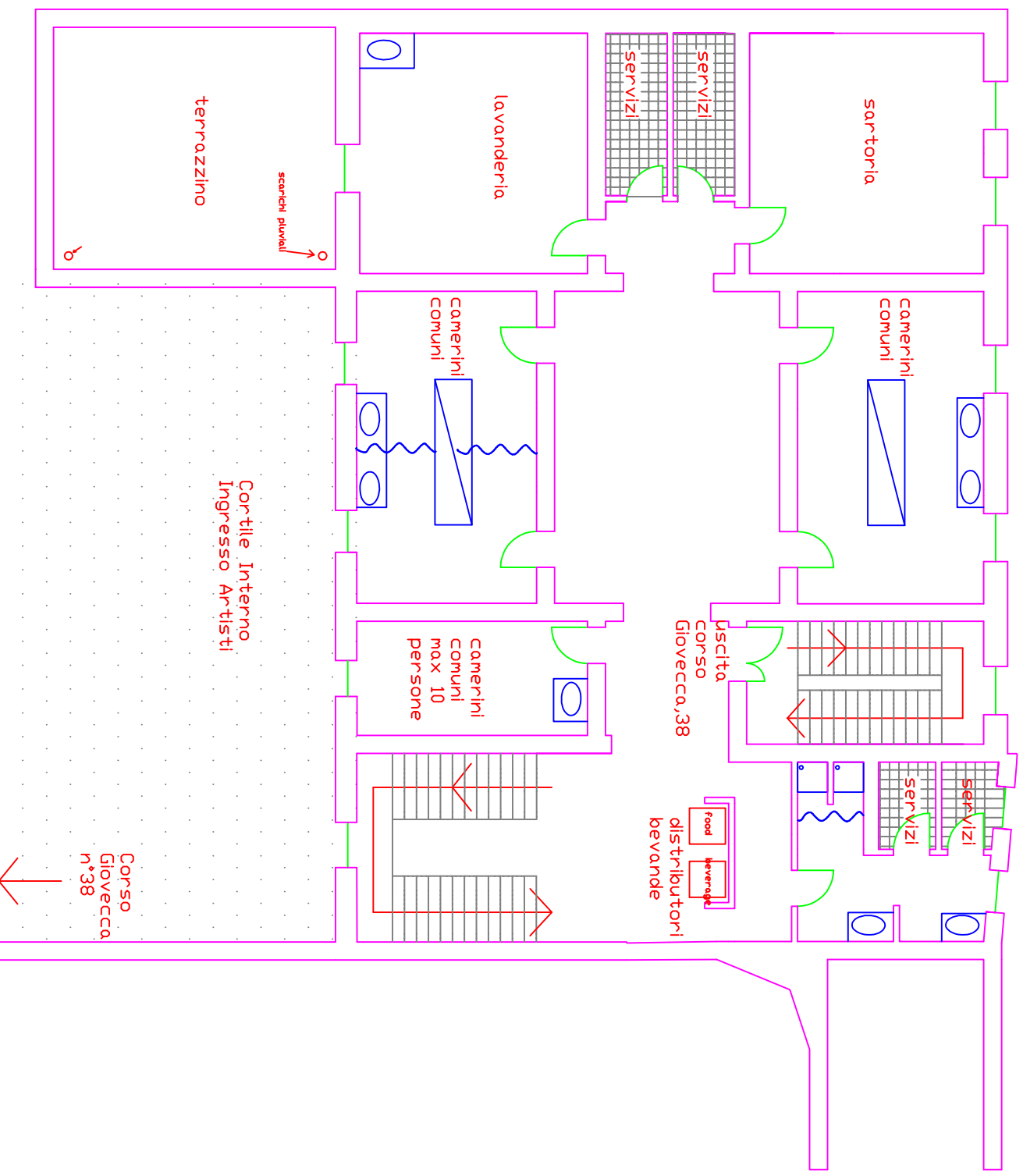
Teatro Comunale di Ferrara-Planimetria Camerini Secondo Piano
